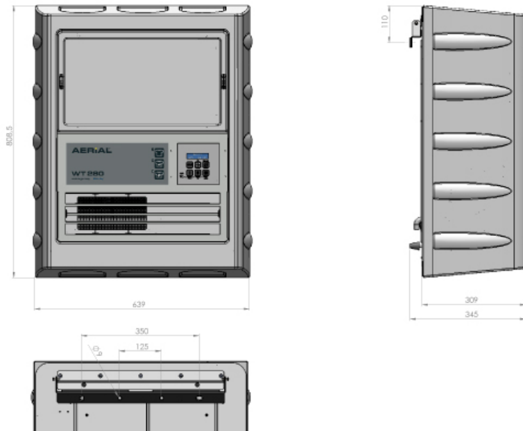
Abb. 2: Maßzeichnung
